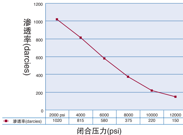
16/30 Interprop 渗透率 (2 lbs/ft 2 @ 250°F)
