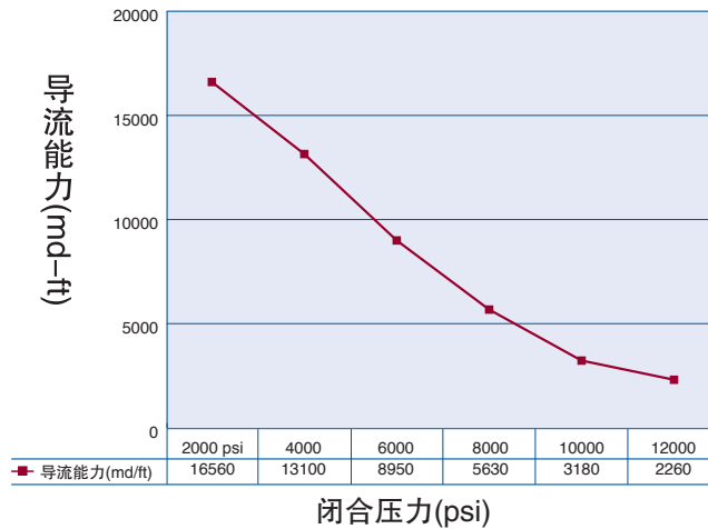
16/30 Interprop 导流能力 (2 lbs/ft 2 @ 250°F)
