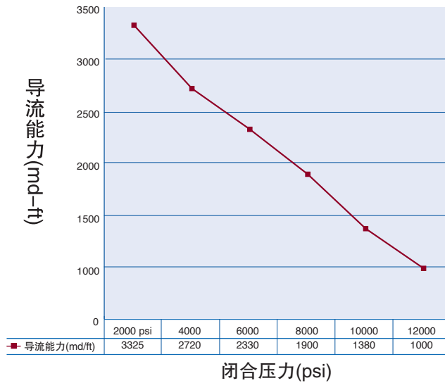
30/50 Interprop 导流能力 (2 lbs/ft 2 @ 250°F)
